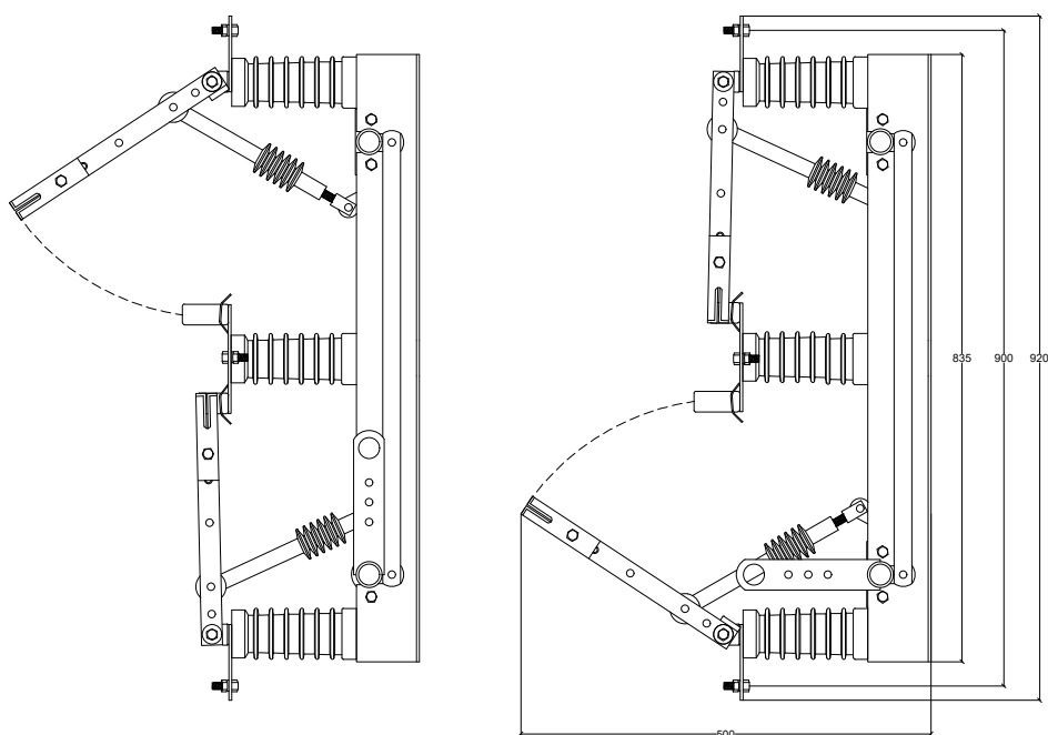
CORTE AA
